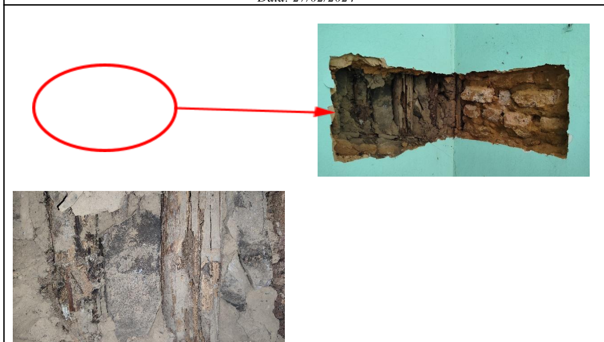
Legenda: Estado de Conservação dos Elementos Estruturais da Alvenaria de Pau-a-pique Autoria: Francielle Ferreira Data: 27/02/2024
