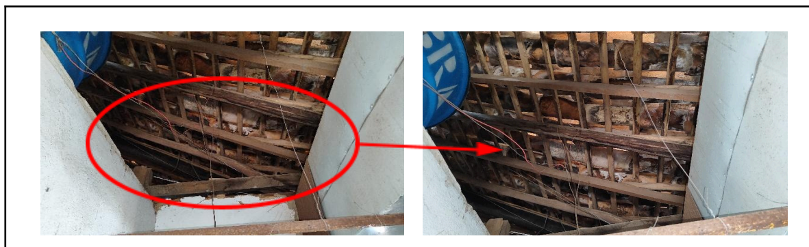
Legenda: Estado de Conservação dos Elementos Estruturais da Cobertura Autoria: Francielle Ferreira Data: 27/02/2024
